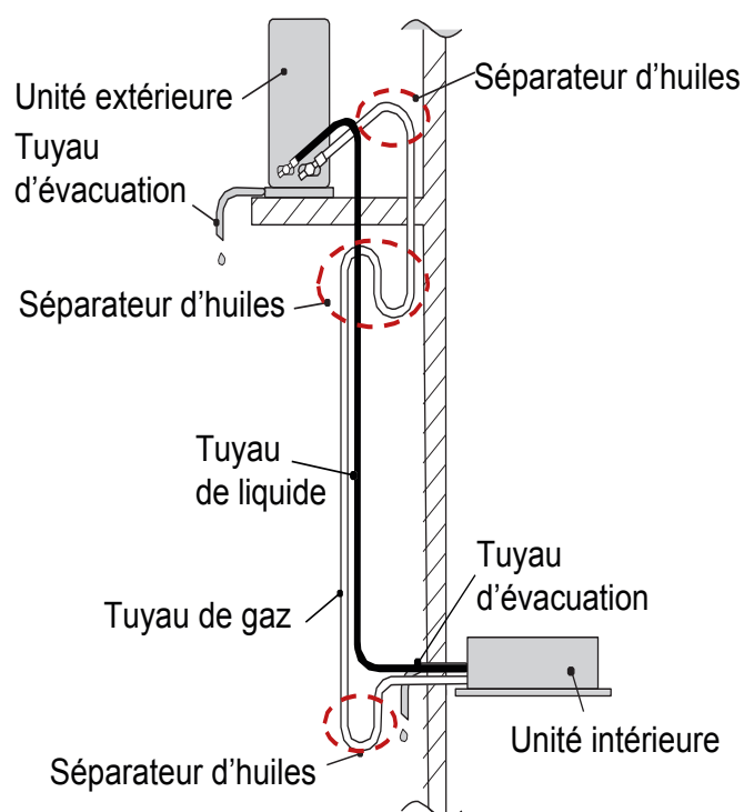
Unité extérieure installée plus haut que l'unité intérieure
