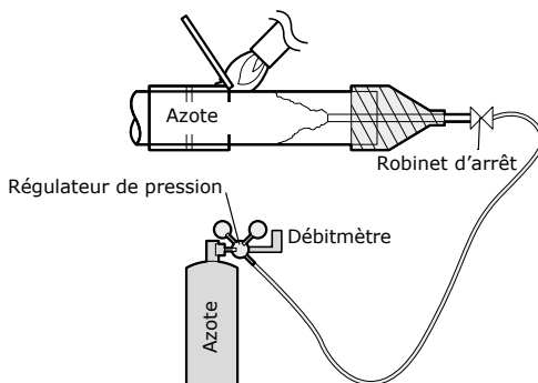
Purge à l'azote lors du brasage des tuyaux de frigorigène
